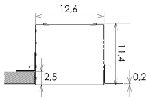
SEZIONE A-A
