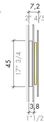
IP 40 TUM 60-T E 2Gx13 40W ED E-ES E-L
